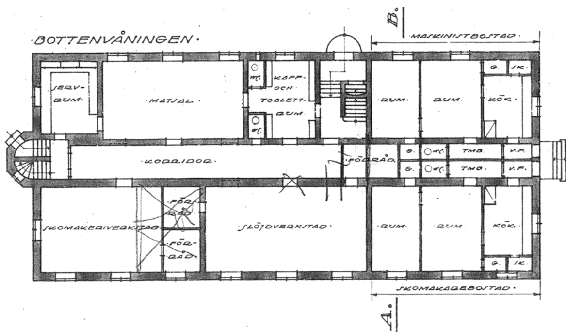
Arbetshem för manliga elever. Ritning, upprättad 1922, på bottenvåningen i C-huset. Samtliga våningsplan finns under Bilagor. Ritningen tillhör Landstingsarkivet.
