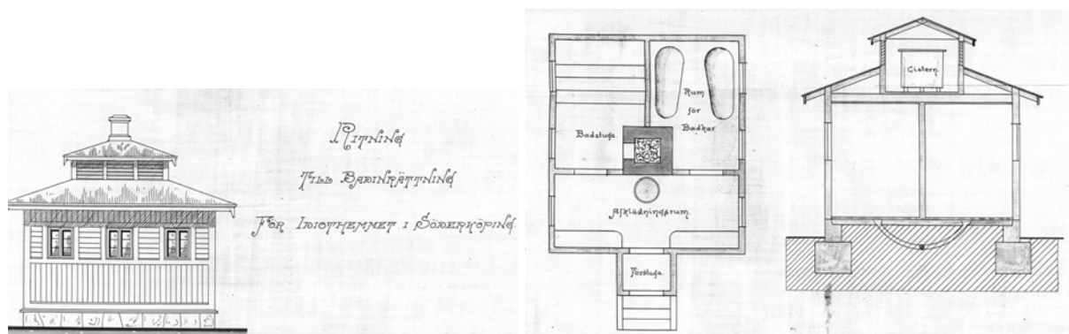
1898 byggdes en badinrättning. Ritningen tillhör Landstingsarkivet.
