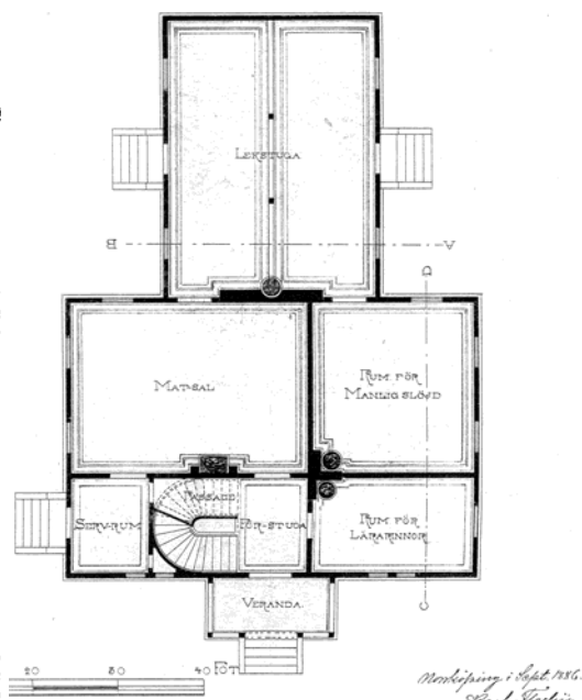
Plan på bottenvåningen.
