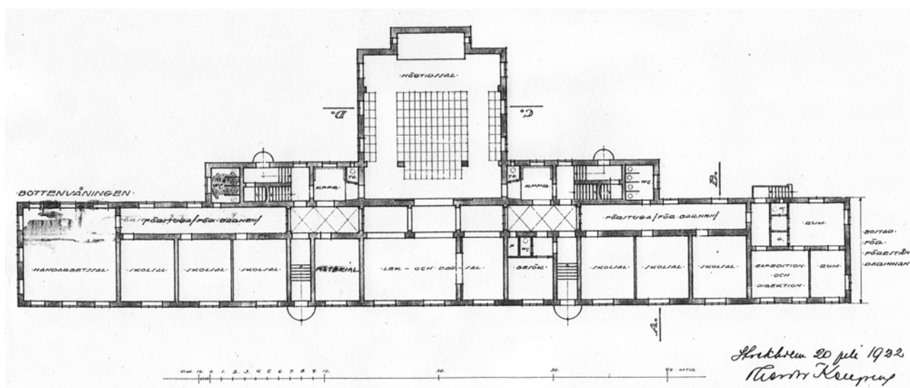
Skolhem. Ritning, upprättad 1922, på bottenvåningen i A-huset. Samtliga våningsplan finns under Bilagor. Ritningen tillhör Landstingsarkivet.
